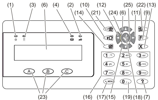
Figuur 2: ATS1135-gebruikersinterface
